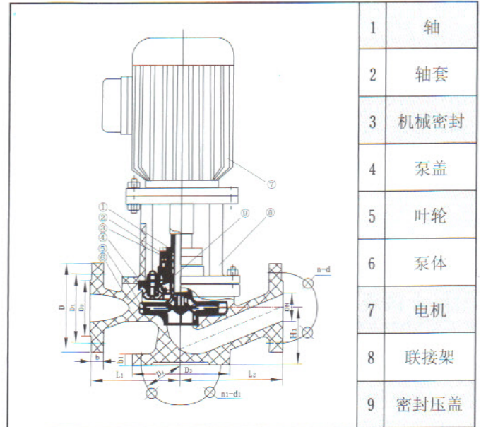
结构图
