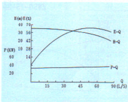
ZW150-180-30
