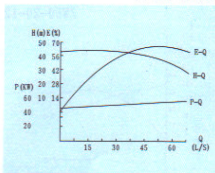
ZW150-180-38
