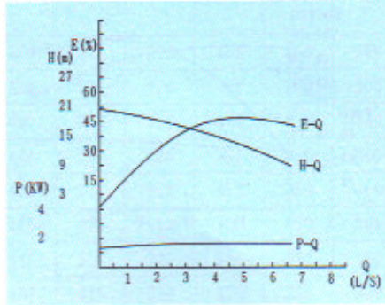
ZW65-30-18 ZW80-40-16
