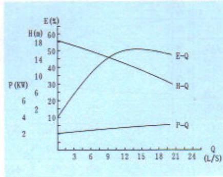
ZW65-30-18 ZW80-40-16
