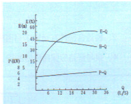
ZW100-100-15
