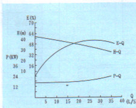
ZW100-100-30
