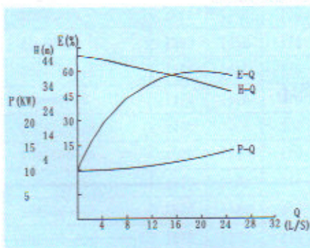
ZW80-80-35
