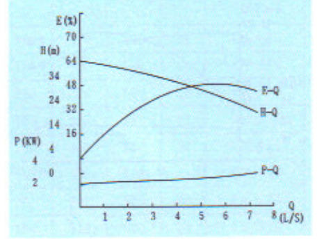
ZW40-15-30 ZW50-15-30
