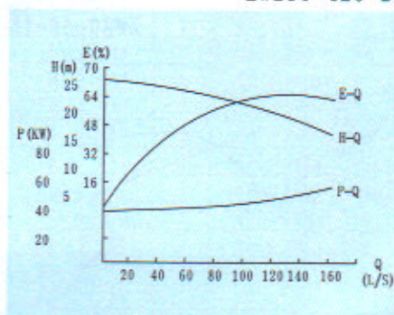
ZW250-420-20
