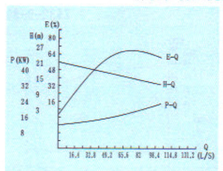
ZW200-280-14
