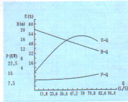
ZW150-180-30
