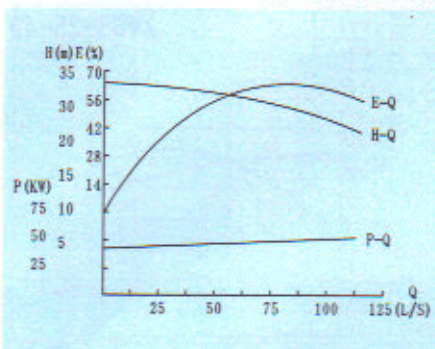
ZW200-280-28
