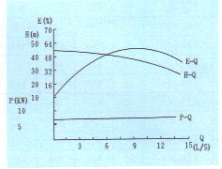
ZW65-25-40
