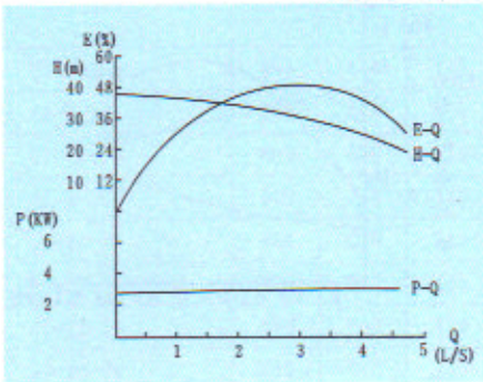
ZW32-9-30
